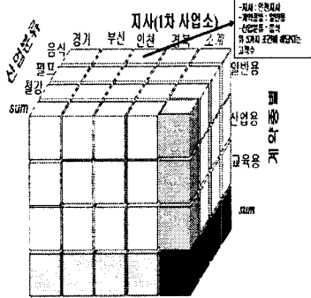
그림 7. 고객분석큐브
