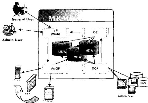
그림 5. 주요처리모듈
