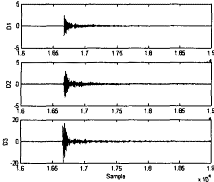
그림 8. 웨이브렛 변환 detail 성분
