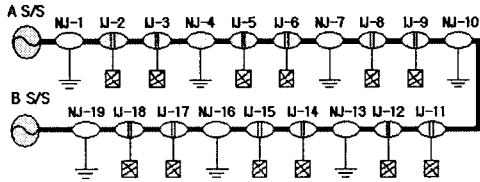
그림 4. 지중송전계통 모델
