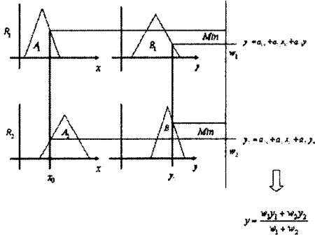
그림 3. 2 입력, 2 규칙 선형추론법
