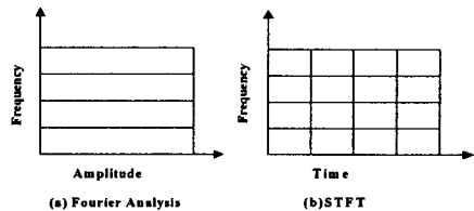
그림 1. 푸리에 변환과 STFT의 신호분석
