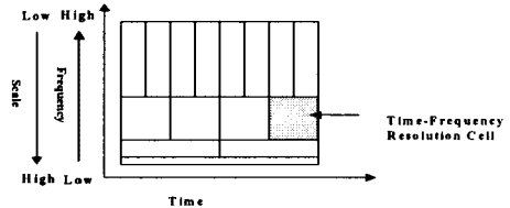
그림 2. 웨이브렛 변환의 시간-스케일의 관계
