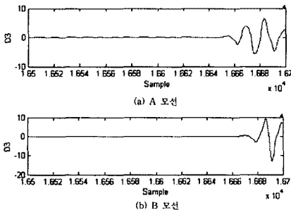
그림 10. D3 성분 확대
