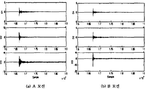
그림 9. 양단 모선에서 측정된 detail 성분 비교
