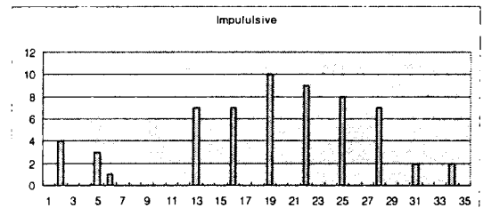
그림 2. Impulsive Transient의 중요벡터 빈도
