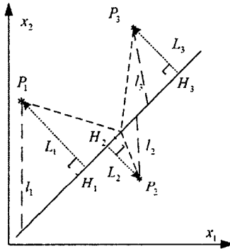
그림 1. 주성분 분석기법의 기본개념
