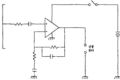
그림2. 저전압 동작형 OP Amp회로
