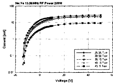
그림 4. 13.56MHz 200W RF 전력에서 Ne:Xe 압력에 따른 I-V 곡선 (semi-log)
