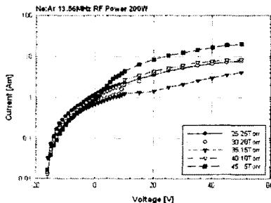
그림 5. 13.56MHz 200W RF 전력에서 Ne:Ar 압력에 따른 I-V 곡선 (semi-log)
