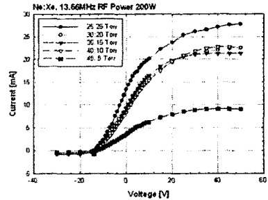
그림 2. 13.56MHz 200W RF 전력에서 Ne:Xe 압력에 따른 I-V 곡선
