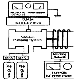
그림 1. 실험장치의 개략도
