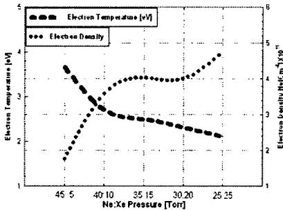
그림 6. 13.56MHz 200W RF 전력에서 전자 온도 및 밀도의 Ne:Xe 압력 의존성
