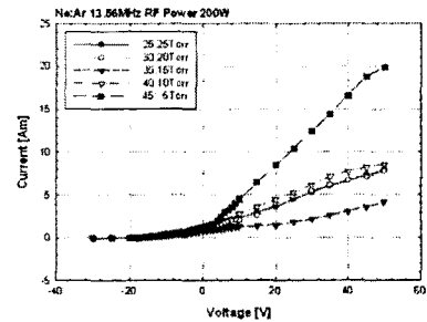
그림 3. 13.56MHz 200W RF 전력에서 Ne:Ar 압력에 따른 I-V 곡선
