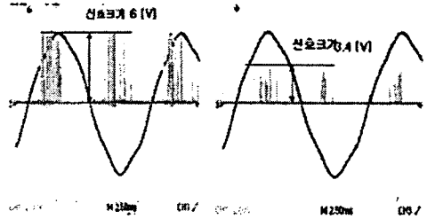
(A) 필터 없는 상태 (B) 30MHz HPF 그림 5. 모의 선로 PD 신호
