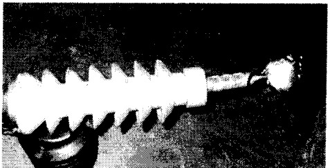
(C) 종단 코로나 방지 처리 그림 1. 모의 선로 제작
