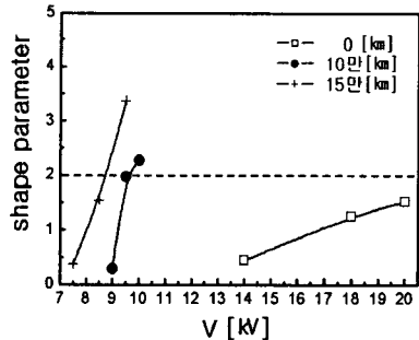
그림 3. 주행거리에 따른 와이블 해석
