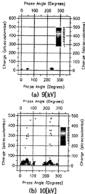
그림 2. 주행거리 10만[km] 점화코일의 \phi-q-n 분포
