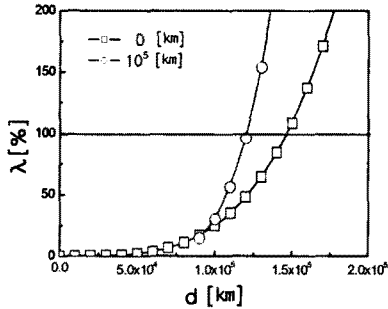
그림 4. 주행거리에 따른 고장률
