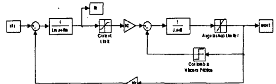
그림 2. 직류모터의 동특성 모델
