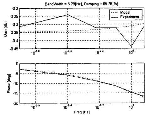
2림 5. 확장 칼만 필터를 이용한 보드선도
