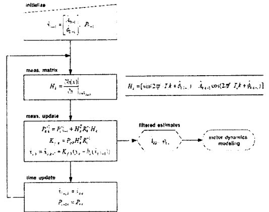
1림 4. 확장 칼만 필터를 이용한 정현파 이득감쇄 및 위상지연 추정
