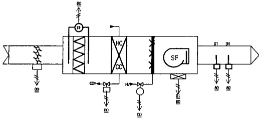
그림 3. 지하층의 자동제어 계통도(정풍량식)
