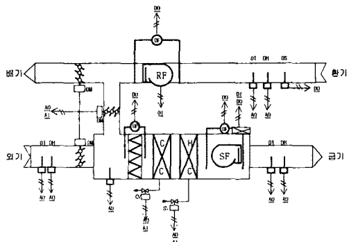
그림 2. 기준층의 자동제어 계통도(정풍량식)
