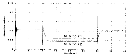
그림 7 슬립에 따른 점착특성
