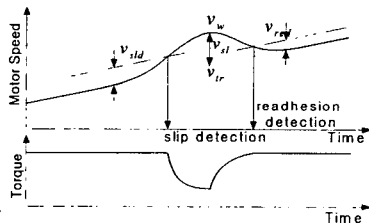
그림 3 슬립제어 패턴
