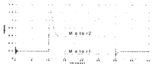
그림 9. 각 전동기축 바퀴 슬립
