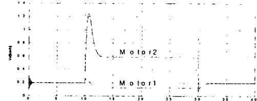
그림 6. 각 전동기축 바퀴 슬립
