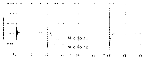
그림 4 슬립에 따른 점착특성
