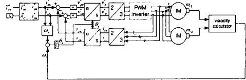
그림 1. 간접벡터제어에 의한 병렬모터구동
