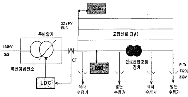
그림 1. 분산형전원이 도입된 배전계통 개념도
