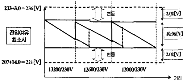
그림 6. 상시전압변동 허용 기준
