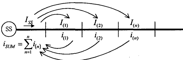
그림 2. 고압배전선의 구간 부하 상징 개념도
