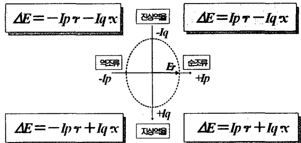
그림 5. 각 상한의 전압강하계산식
