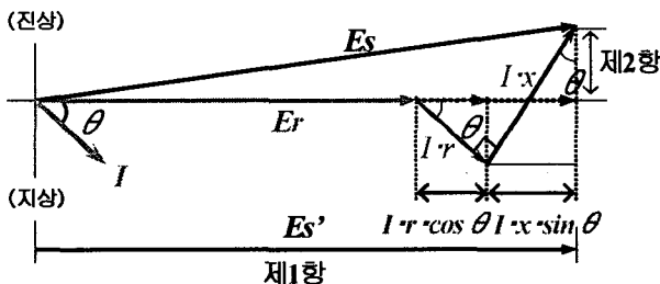
그림 3. 일반적인 전압강하 계산식
