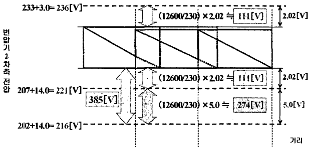
그림 7. 순시전압변동 허용 기준
