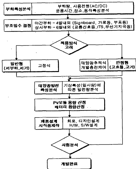
그림 1 소규모 태양광 발전시스템의 설계흐름도
