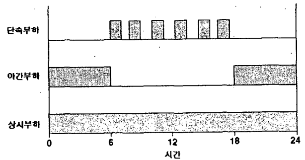
그림 2 독립형 태양광 발전시스템의 부하특성
