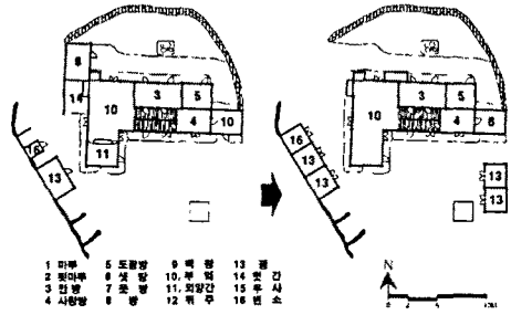
<그림 2-3> 함병식 가옥 평면도
