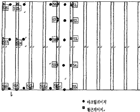
Fig. 2 게이지 부착 위치
