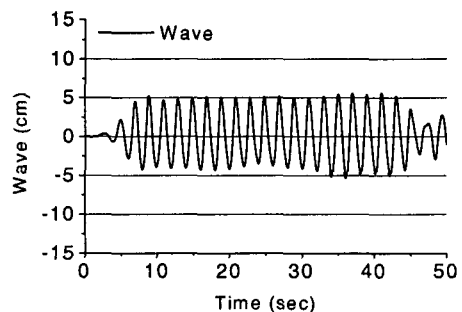
Fig. 3 파고
