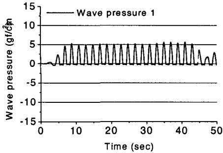
Fig. 4 파압 A
