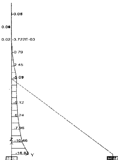
Fig. 9 중앙말뚝 모멘트
