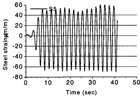
Fig. 6 S5 위치에서의 철근 변형률
