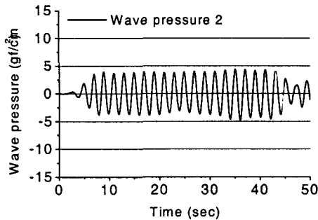
Fig. 5 파압 B
