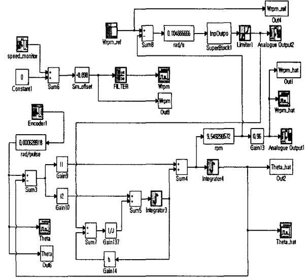
그림 5 속도관측기를 사용한 속도제어기 설계 Fig. 5 Design of speed controller using speed observer
