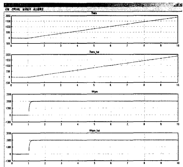
그림 6 속도관측기를 사용한 속도제어기 응답 Fig. 6 Response of speed controller using speed observer
