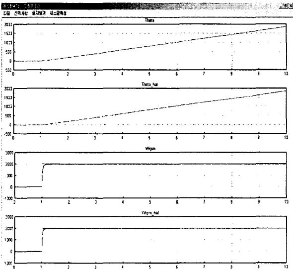
그림 4 엔코더 속도제어기에 의한 속도관측기 응답 Fig. 4 Response of speed observer by speed controller using encoder
