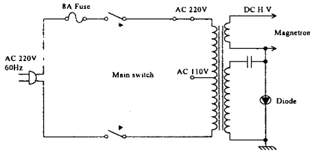
그림 2. 마이크로파 발진용 전원회로
