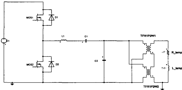
그림 4. 시뮬레이션도 회로 Fig. 4. Simulation circuit
