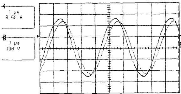
그림 11. 램프의 전압, 전류 실험 파형(1usec/div) Fig. 11. Experiment waveform of lamp voltage/current
