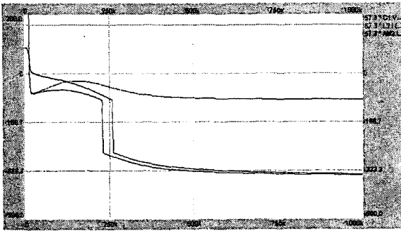
그림 9. 필터의 주요 성분의 위상특성 Fig. 9. Filter phase characteristics
