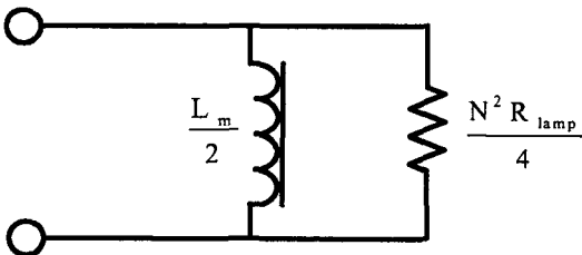
(b) 병렬 등가 회로
