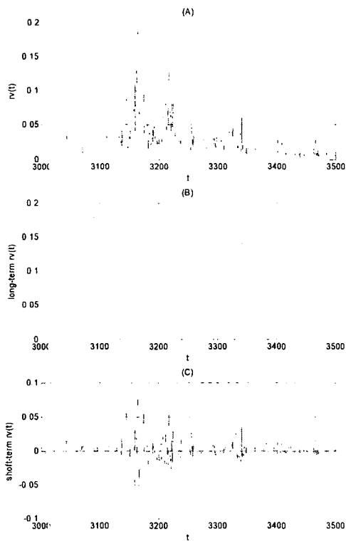
그림-1: 소파동을 이용한 장기,단기 변동성 분해, t=3000, 3500 (A) 실현변동성 (B) 장기변동성 (C) 단기변동성
