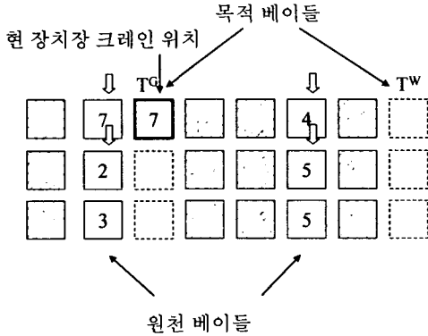
그림 8. 컨테이너 7G를 옮긴 직후의 블록 상태
