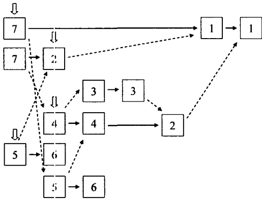
그림 7. 컨테이너 7G를 옮긴 직후의 이동 순서 제약
