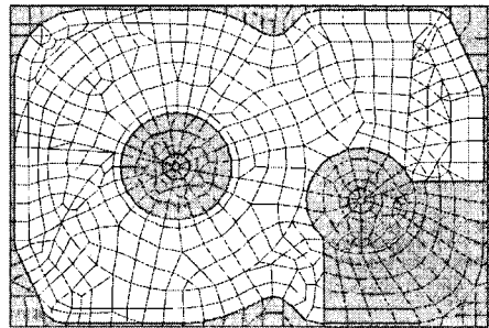
Fig 4. 디자인 대상 영역
