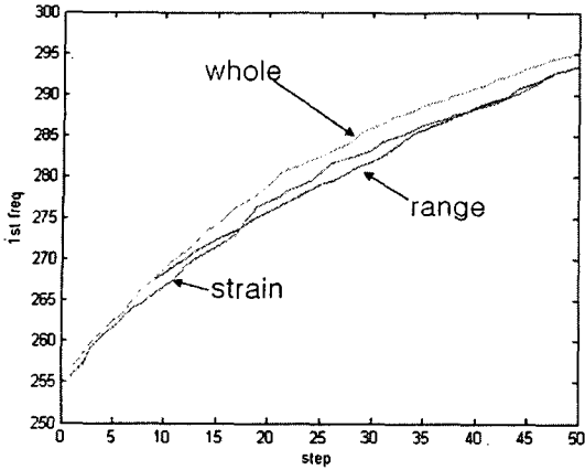
Fig 5. 1차 고유진동수
