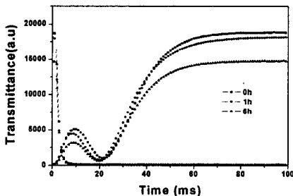
그림 3. 폴리이미드 표면을 이용한 3종류의 TN 셀의 응답특성.
