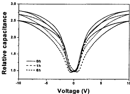
그림 4. 광폴리머 표면을 이용한 광배향 TN-LCD의 C-V 특성.
