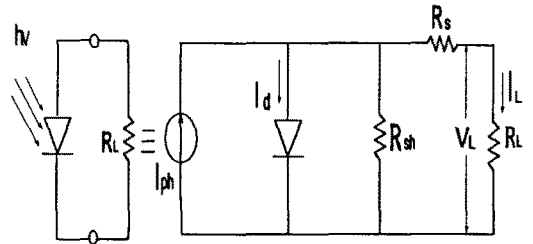
Fig. 1 태양전지 등가회로
