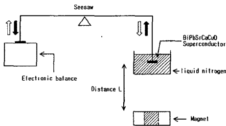
그림 2. 자기력 측정장치
