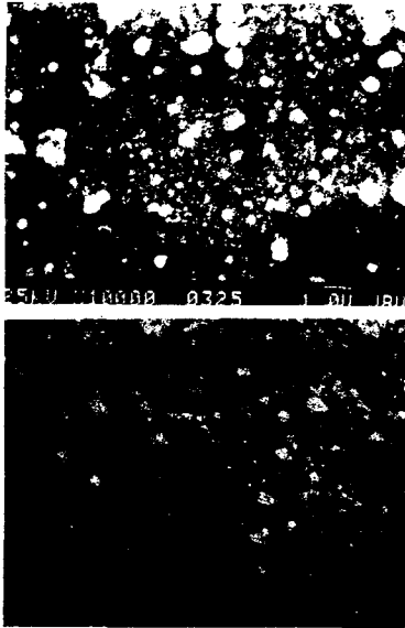
그림2. CBD-CdSe 박막의 표면형상: 열처리하지 않음(위), 450°C에서 열처리(아래)
