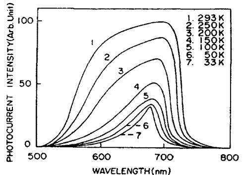
그림 5. 450°C에서 1시간 열처리한 CBD-CdSe 박막의 광전류 스펙트럼
