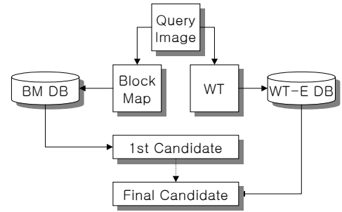
그림 2. 제안한 시스템 구조도
