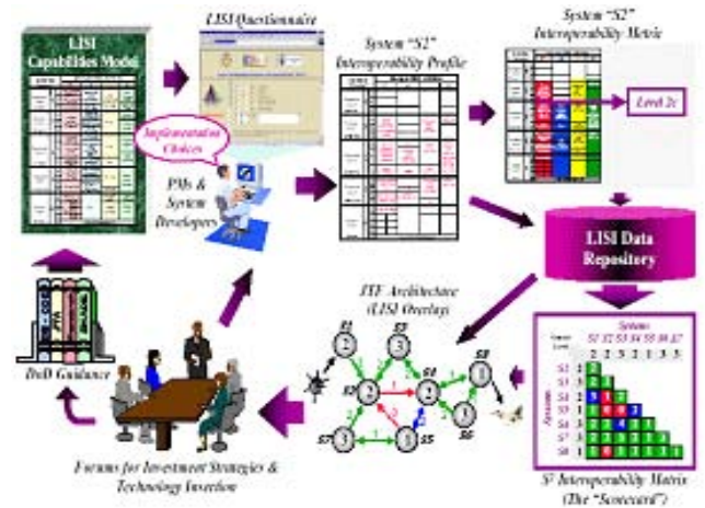
(그림 2) LISI 심사 프로세스[2]
