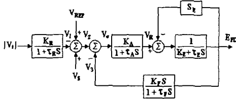
그림 2. IEEE Type 1 여자기 블록선도
