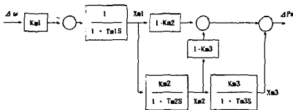
그림 3. 조속기 블록선도
