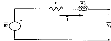
그림 1. 발전기 이축모델의 등가회로
