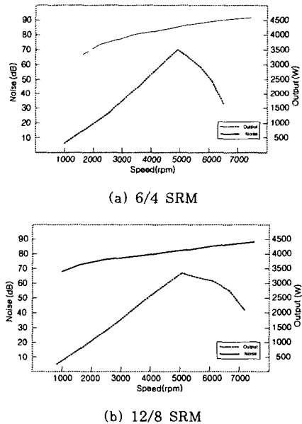
그림 6. 피시험 전동기의 소음측정 Fig. 6. Noise measurement of prototype SRM
