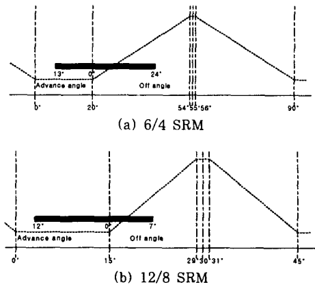
그림 5. 피시험 전동기의 인덕턴스 프로파일과 스위칭 각도 (5000rpm일 때) Fig. 5. Inductance profiles and switching angle of prototype SRM(at 5000rpm)
