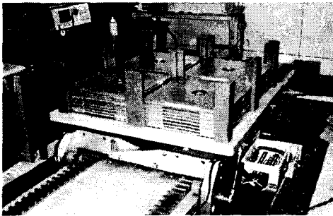
그림 7. 제작된 CPM형 자기부상 반송 시스템
