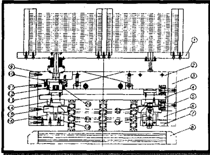
그림 6 CPM형 자기부상 시스템의 도면
