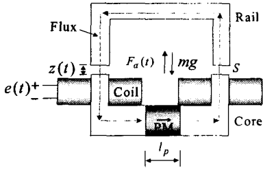
그림 1 CPM 자기부상 시스템
