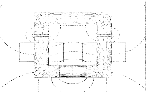
그림 3 전자장 해석 결과 : 자속 패턴
