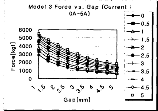
그림 4 공극, 전류 및 부상력 특성곡선
