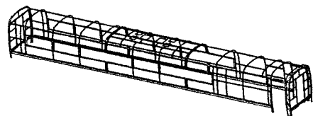
그림 8. 복합재 차체내의 삽입 골조
