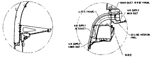
(a) 금속재 차량
