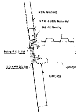
그림 7. 복합재 차체와 언더프레임과의 체결 방법
