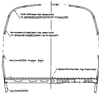
그림 4. TTX 하이브리드 복합재 차체 단면
