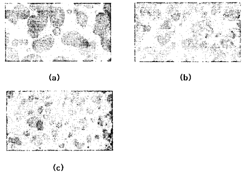
Fig. 2 가열온도 60, 70, 80℃가 적용된 최종 제품 단면의 미세형상: a) 가열온도 60℃ b) 가열온도 70℃ c) 가열온도 80℃. 당김속도와 발포제 함유량은 각각 9.5mm/min과 3wt%임.
