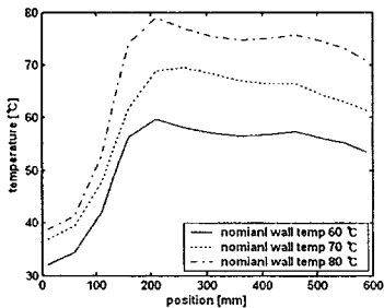
Fig. 1 열전대로 측정된 실제의 다이 내부 온도분포. nominal wall temp는 설정한 가열 온도를 말한다.
