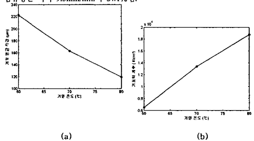
Fig. 3 가열온도 60, 70, 80℃가 적용된 최종 제품의 기포 평균 직경과 기포의 개수 추이: a) 기포 평균 직경 b) 기포의 개수. 당김속도와 발포제 함유량은 각각 9.5 mm/min과 3wt%임.
