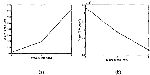
Fig. 7 발포제 함유량 1, 3, 5wt%가 적용된 최종 제품의 기포 평균 직경과 기포의 개수 추이: a) 기포 평균 직경 b) 기포의 개수. 가열온도와 당김 속도는 각각 80℃와 9.5mm/min임.
