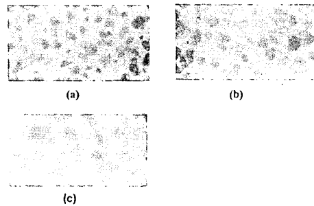
Fig. 6 발포제 함유량 1, 3, 5wt%가 적용된 최종 제품 단면의 미세 형상: (a) 발포제 함유량 1wt% (b) 발포제 함유량 3wt% (c) 발포제 함유량 5wt%
