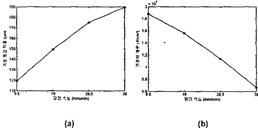
Fig. 5 당김 속도 9.5, 19.0, 28.5, 38.0mm/min가 적용된 최종 제품의 기포 평균 직경과 기포의 개수 추이: a) 기포 평균 직경 b) 기포의 개수. 가열온도와 발포제 함유량은 각각 80℃와 3wt%임.
