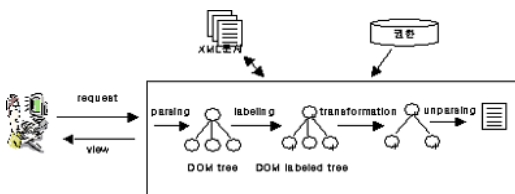
▶▶ 그림 2. XML 문서의 접근 제어 수행 과정
