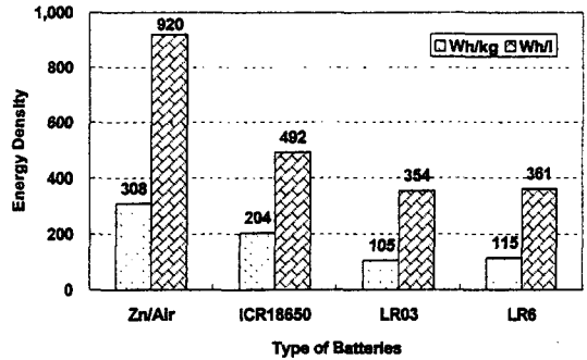
그림 10 타 전지와 에너지밀도 비교 Fig. 10 Comparison of energy density with other batteries
