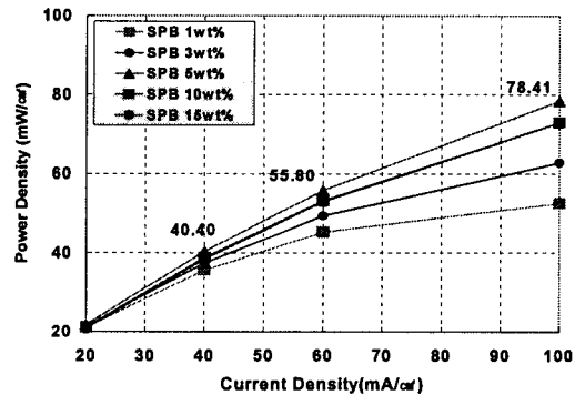
그림 6 도전재 함량에 따른 전지의 출력특성.
