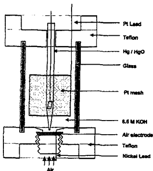
그림 3 Half Cell 구조. Fig. 3 Structure of Half cell.
