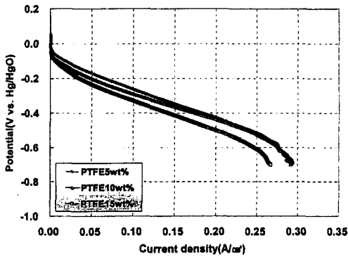
그림 8 양극 내 PTFE 함량에 따른 방전을별 전지성능 Fig. 8 Variations of cathode performance according to contents ratio of binder.
