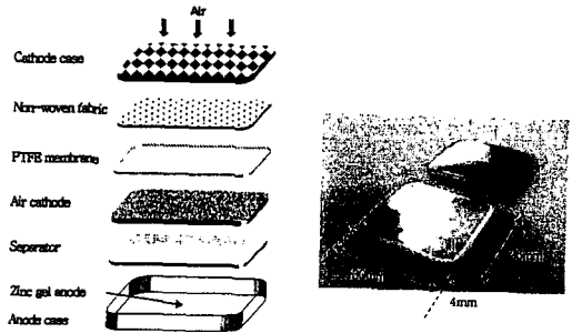
그림 4 단위전지 개략도. Fig. 4 Schematic drawing of unit cell.
