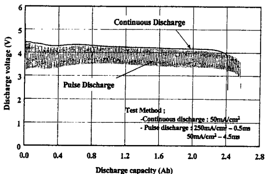
그림 13 아연공기 전지팩의 펄스방전성능
