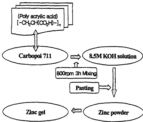
그림 2 음극제조과정 Fig. 2 Manufacturing process of Anode.
