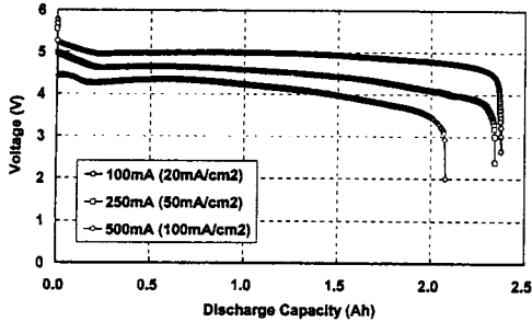
그림 12 아연공기 전지팩의 전류밀도별 방전 성능
