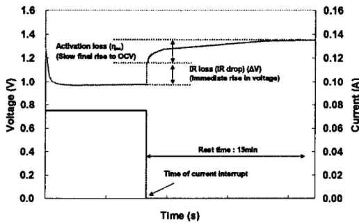
그림 5 Current interrupt 방법에 의한 전압, 전류 거동.
