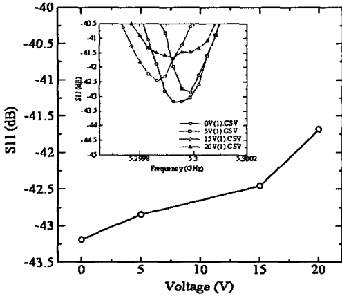
그림 4. 유기발광소자내의 인가전압에 따른 반사계수 S_{11} .
