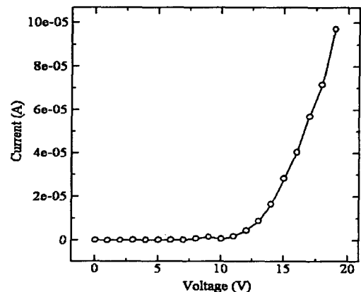
그림 3. 유기발광소자의 전류-전압 특성.
