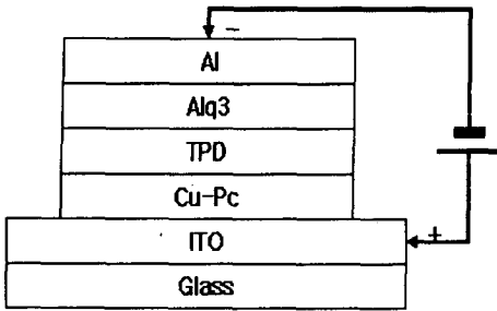
그림 1. 실험에 사용한 소자의 구조. Fig 1. Typical device structure.
