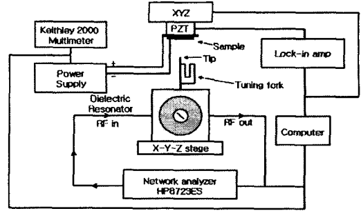
그림 2. 유전체 공진기를 사용한 실험 배열 구조도. Fig 2. Diagram of the experimental configuration with a dielectric resonator.
