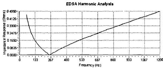
그림 10. 임피던스 응답특성 Fig. 10. Impedance response characteristic
