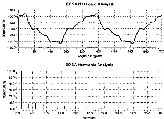
그림 12. 선로 전류 파형 Fig. 12. Branch current waveform
