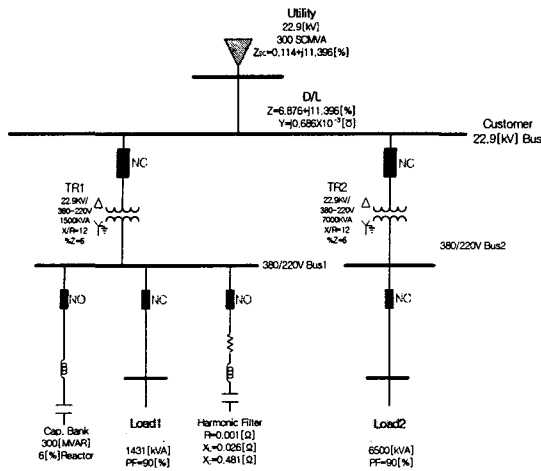
그림 1. 사례연구 배전시스템 Fig. 1. Single-line diagram of the distribution system under study
