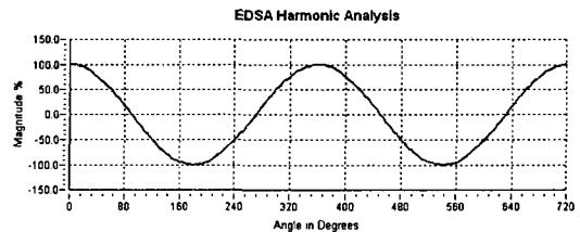
그림 4. 22.9(kV) 모선 전압파형 Fig. 4. 22.9(kV) Bus voltage waveform
