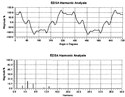
그림 3. 고조파 발생 전류 파형 Fig. 3. Load current waveform
