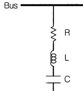
그림 9. 수동 동조 필터 Fig. 9. Passive resonant filter
