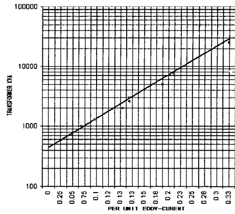
그림 6. 변압기 정격과 와류손의 관계 Fig. 6. Relationship between Transformer rating and Eddy-current
