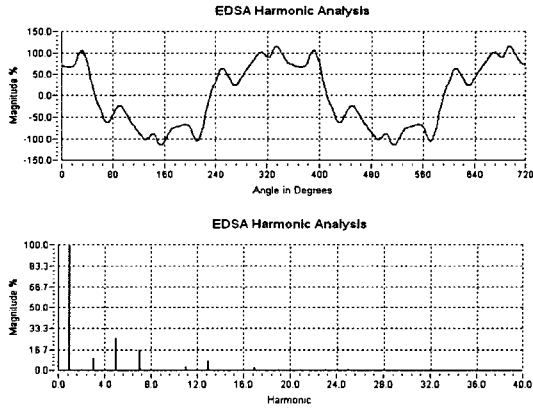
그림 5. 선로 전류파형 Fig. 5. Branch current waveform
