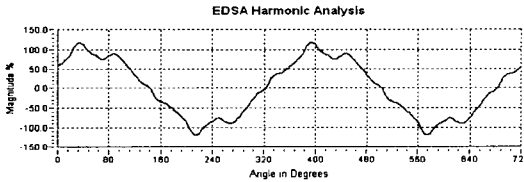
그림 9. 수동 동조 필터 Fig. 9. Passive resonant filter
