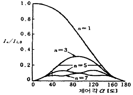
그림 3-2 전력조정기의 고조파 전류
