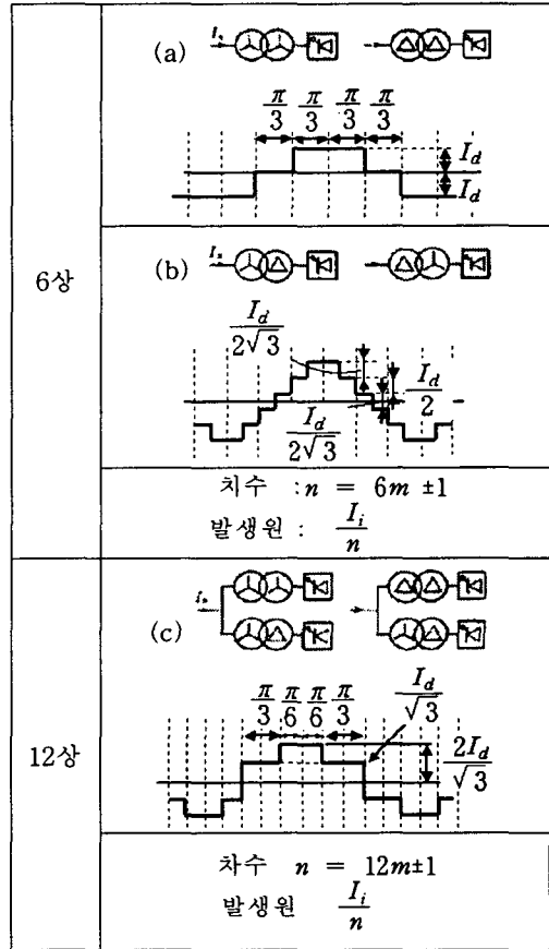
그림 3-5 3상 정류기의 교류측 전류파형
