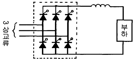
그림 3-4 6상 전력 변환장치
