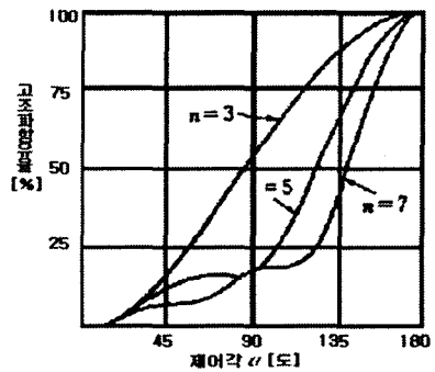
그림 3-3 고조파 전류 함유율
