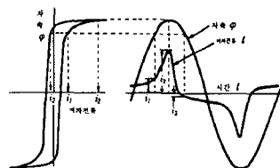
그림 3.7 여자 전류 파형
