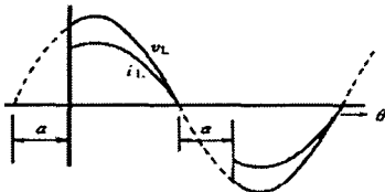
그림 3-1 전력조정기에 의한 전압전류파형
