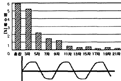
그림 3-6 콘덴서 입력형 전원 회로의 기기에 의한 전압 외형
