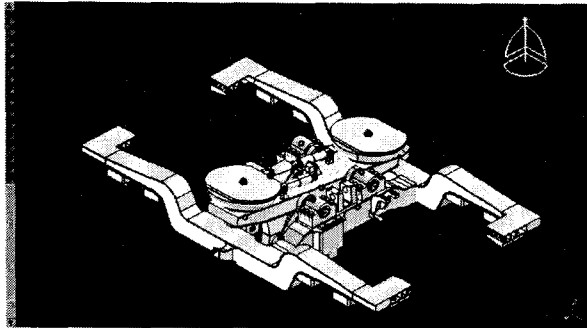
그림 6 TTX_PDM을 이용한 3D 대차 모형제작
