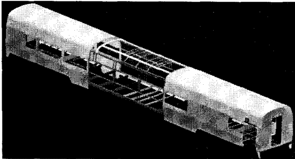
그림 5 TTX_PDM을 이용한 3D 차체 모형제작
