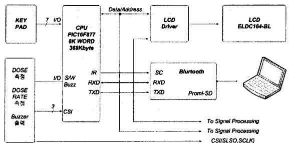
그림 4. 제어부 구성도
