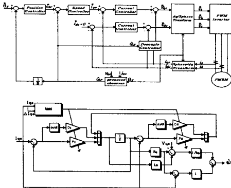
그림 3.1 (a) 시스템 전체 구성도 (b) 제안된 시스템의 블록선도 Fig. 3.1 (a) Total Structure of System (b) Block diagram of the Proposed system
