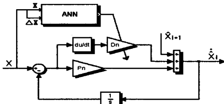
그림 2.1 뉴로 관측기의 구조
