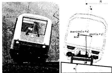
그림 1 틸팅차량의 횡가속도 저감의 원리
