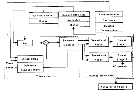
그림 6. 틸팅제어 블록도
