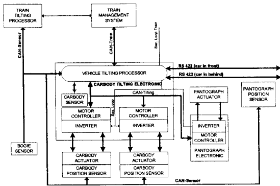
그림 4. 틸팅차량 인터페이스 블록도
