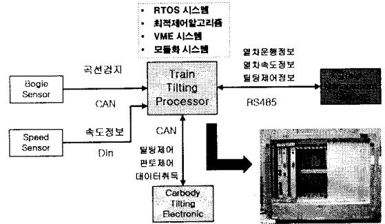
그림 5. 틸팅제어장치 블록도
