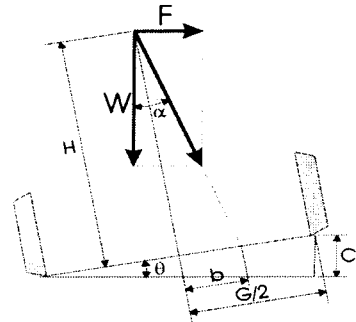
그림 2 곡선부 원심력과 중력의 합력관계
