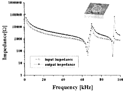
그림 3. 압전 변압기의 임피던스 해석
