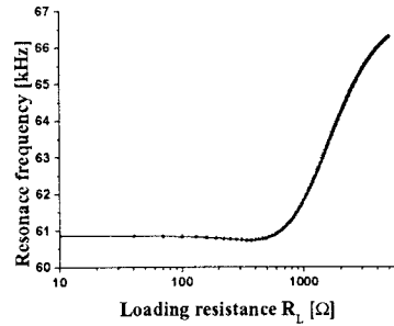
그림 5. 부하에 따른 공진 주파수의 변화
