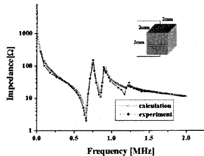
그림 2. 임피던스 파형의 비교
