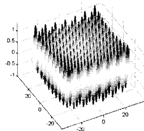
그림 7. 시험 함수
