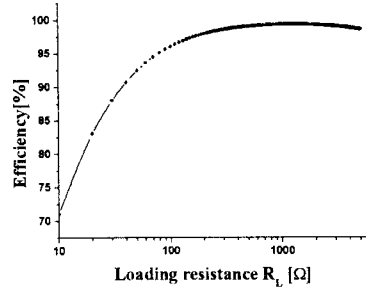
그림 6. 부하에 따른 효율의 변화
