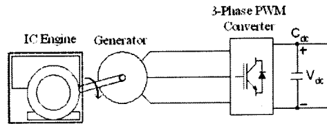
그림 2. 발전기 계자시스템
