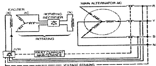
그림 1. 발전기 계자시스템
