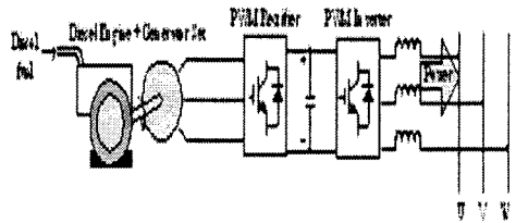
그림 4. 디젤엔진 발전기를 이용한 계통연계시스템 전체블록다이어그램
