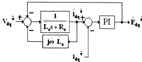
그림 3. 역기전력 추정방법
