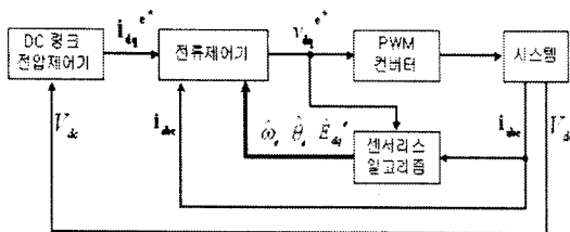
그림 4. PWM제어 전체 블록도
