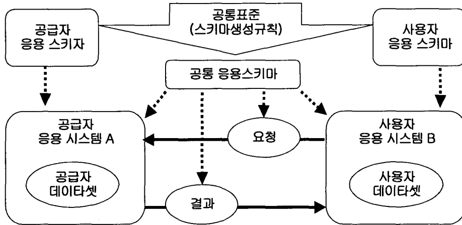
그림 1. 공통응용스키마에 의한 데이터교환
