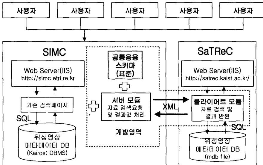
그림 2. 그리드데이터 메타데이터 통합검색시스템 구조도
