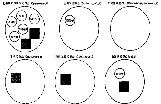
그림 3 KRISTAL-2002 JAVA API 파라미터 클래스들
