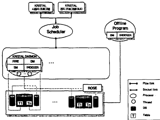
그림 1 KRISTAL-2002 시스템의 구조
