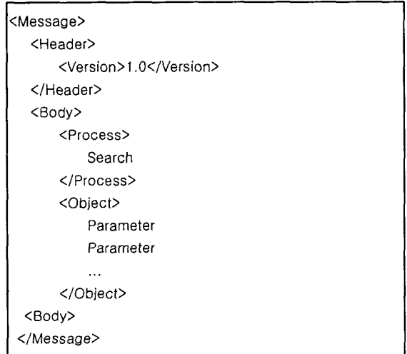
그림 2 KRISTAL-2002 XML 메시징 프로토콜 구조
