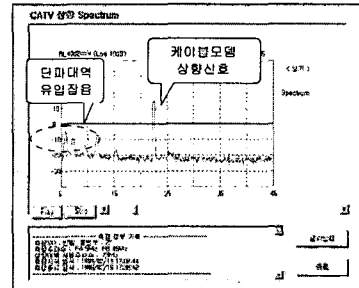
그림 2. 대표적인 상향대역 신호 유형
