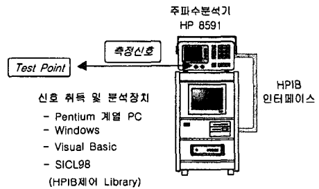
그림 1. 상향대역 신호 측정 데이터 취득분석 장치 구성도
