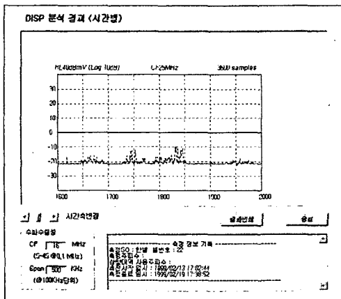
그림 4. 한밭SO 시간별 신호레벨 변화
