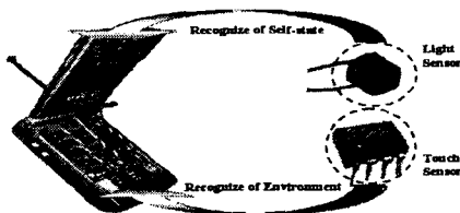
그림 7. 감성추론엔진의 구성
