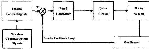
그림 5. 감성발향 모듈의 제어 시스템
