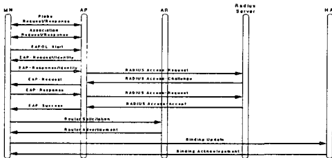
그림 4. MIPv6를 이용한 WLAN 접속 절차
