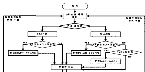
그림 2. 로밍 결정 과정 순서도
