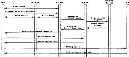
그림 3. MIPv6를 이용한 3GPP망 접속 절차
