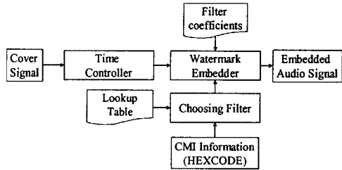
그림 3. 워터마킹 삽입 시스템
