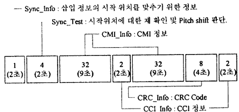
그림 1. Payload 구조
