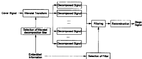
그림 2. 정보 삽입 구조도
