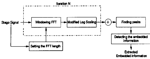
그림 4. 삽입 정보 추출 구조
