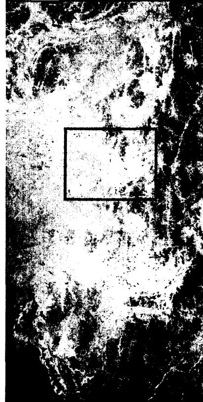
그림 7. KH-9 영상 2
