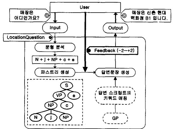
그림 2. 답변 생성의 구조
